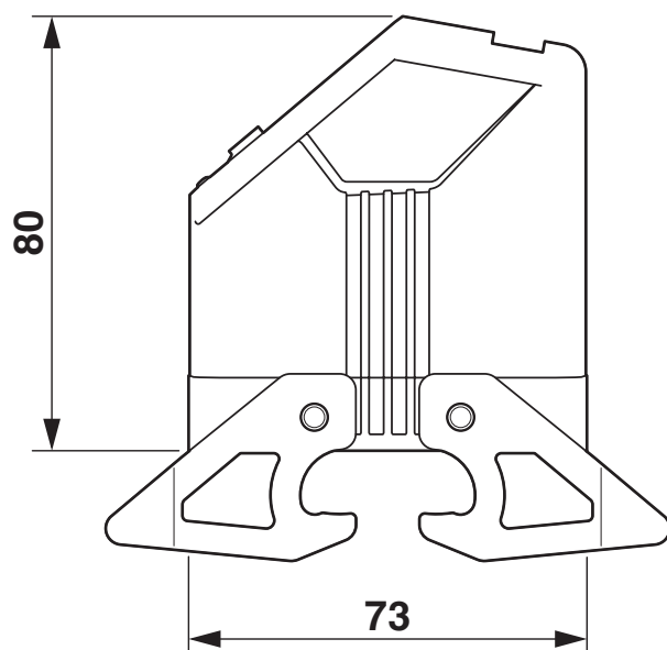
Dessin coté
