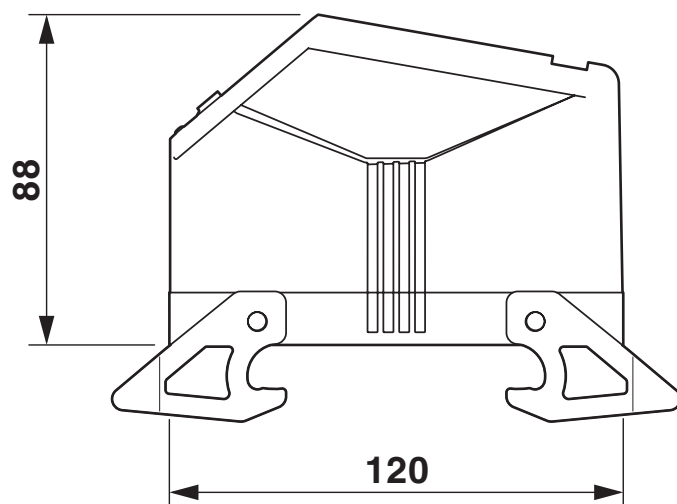
Dessin coté
