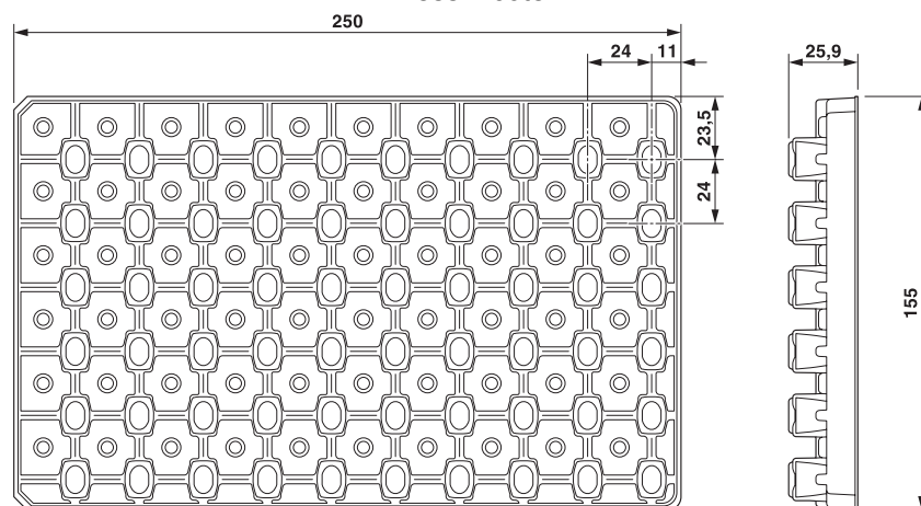
Dessin coté
