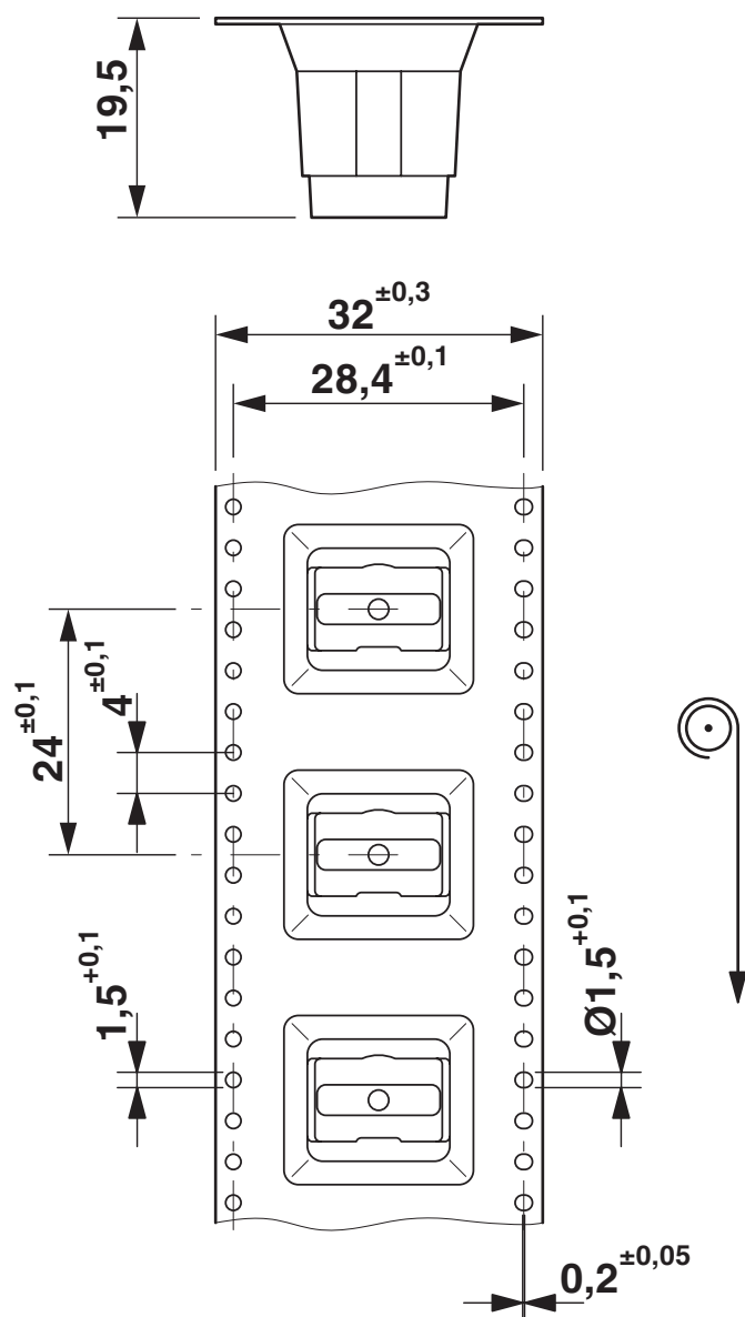
Dessin coté
