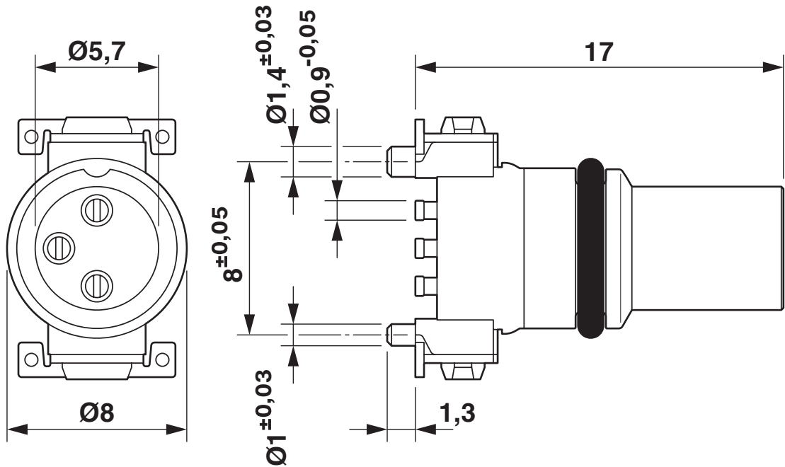
Dessin coté
