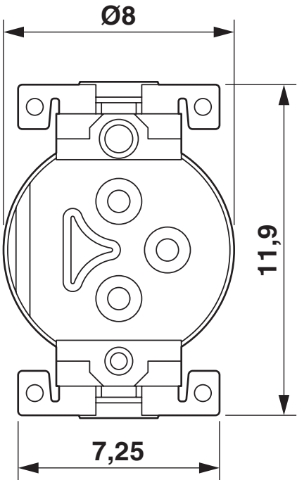
Dessin coté
