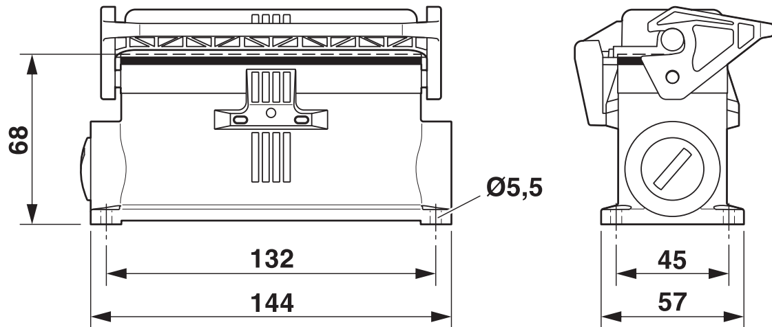
Dessin coté
