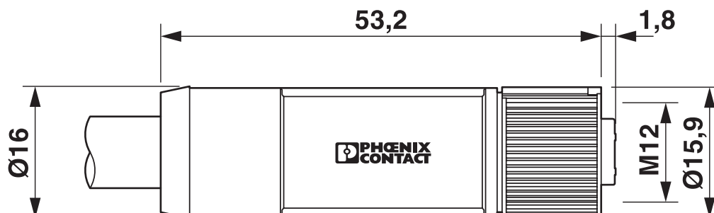
Dessin coté
