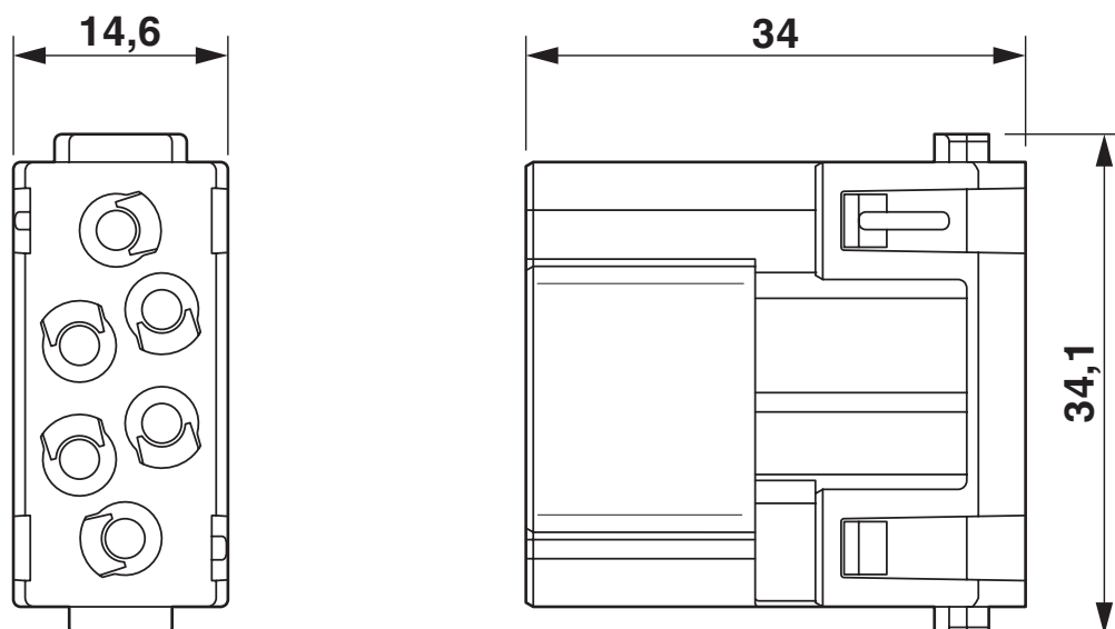
Dessin coté
