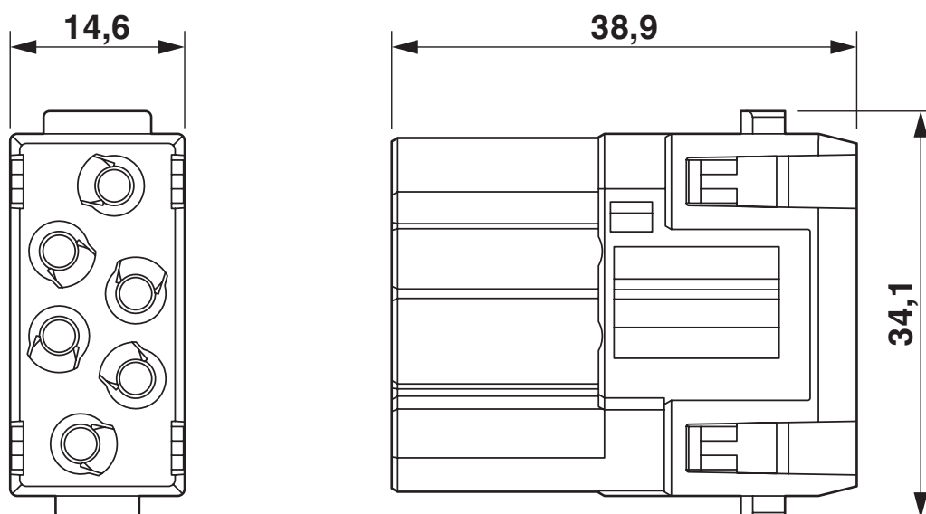
Dessin coté
