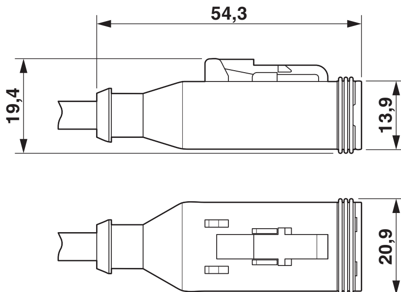
Dessin coté
