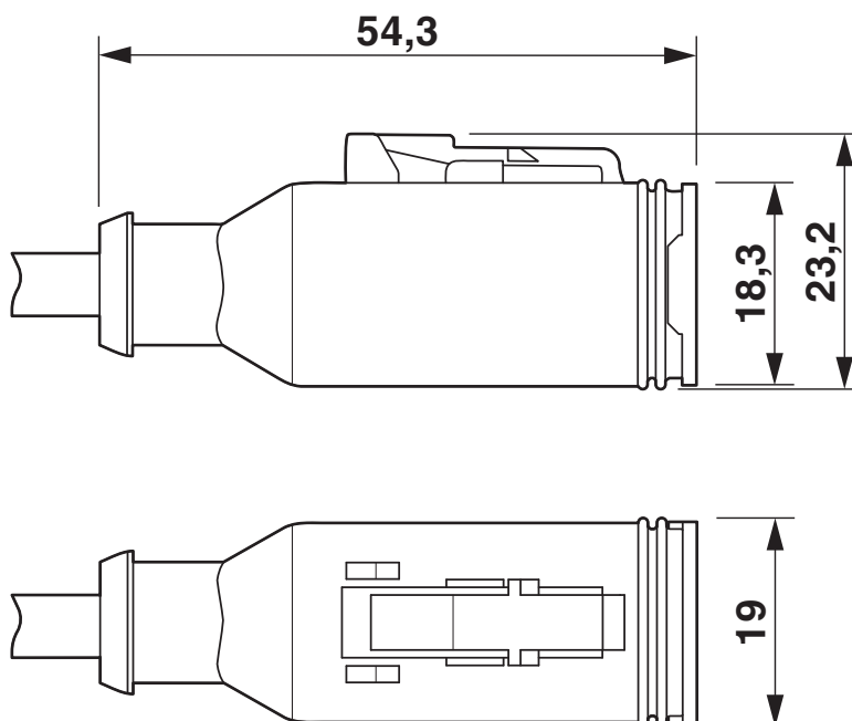
Dessin coté
