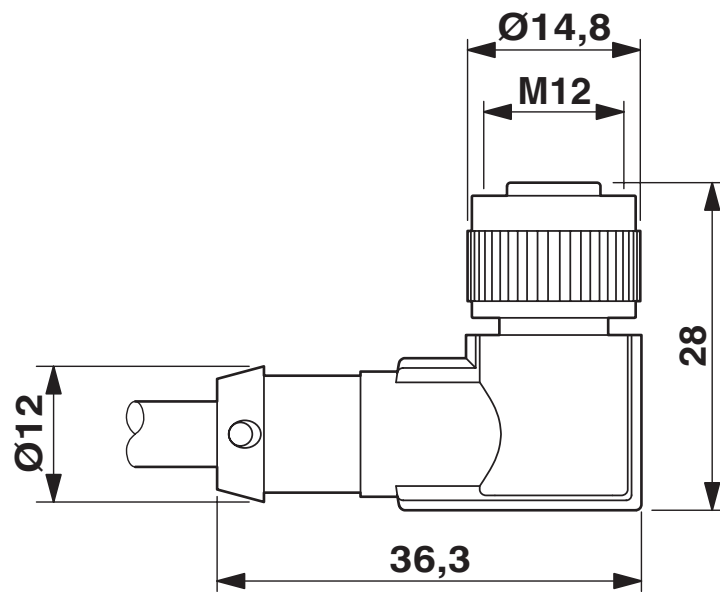
Dessin coté
