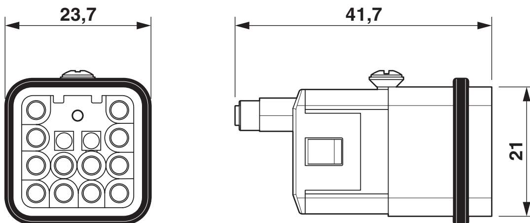
Dessin coté : HC-Q 12-I-CT-M
