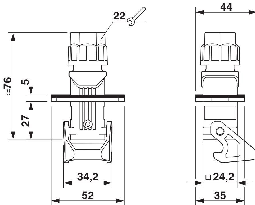
Dessin coté
