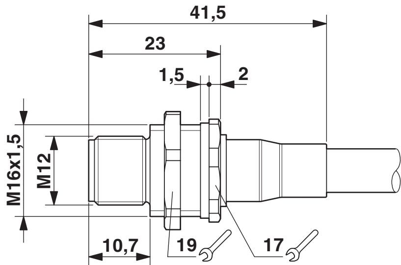
Dessin coté
