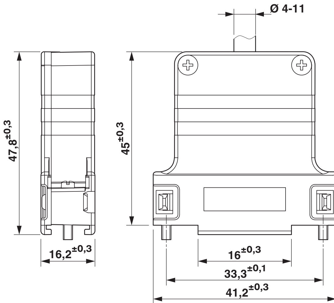
Dessin coté
