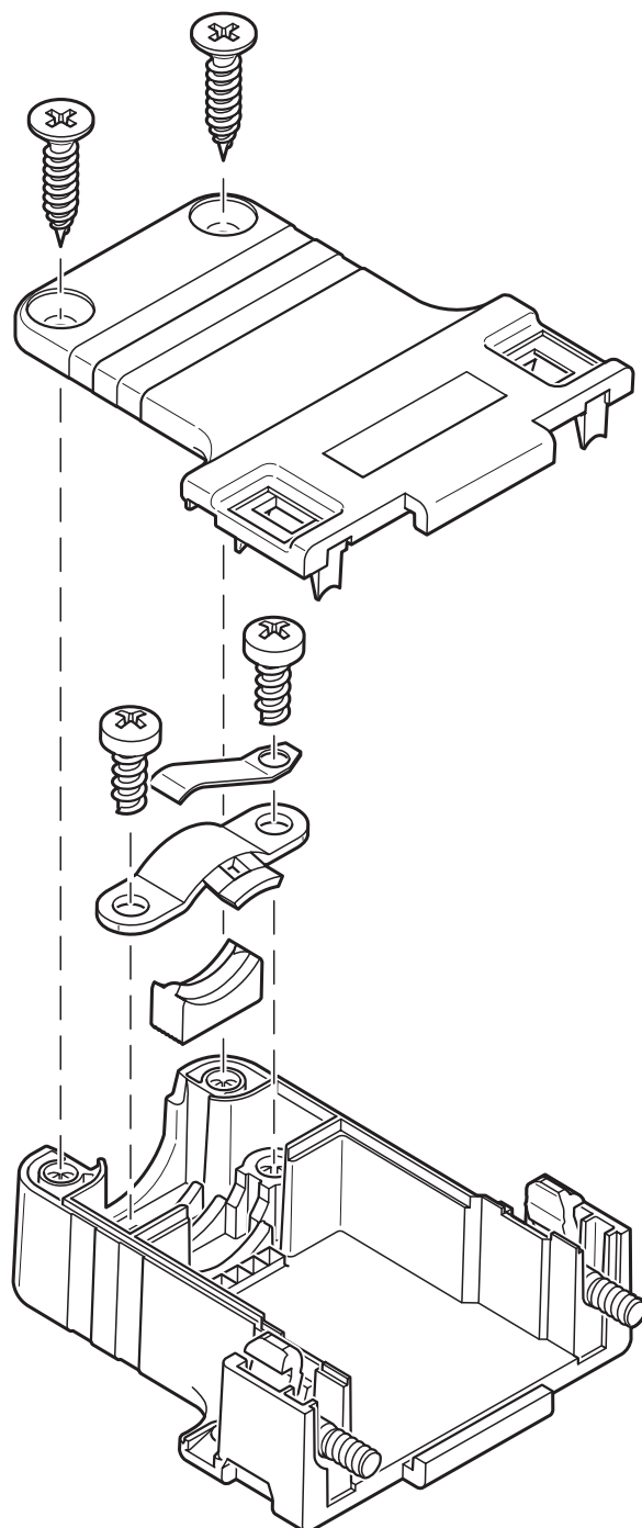
Dessin schématique
