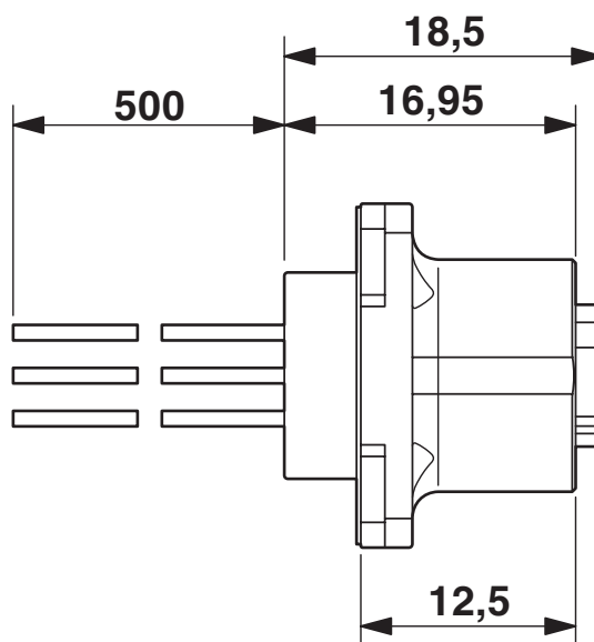
Dessin coté
