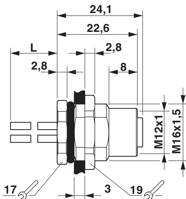
Dessin coté
