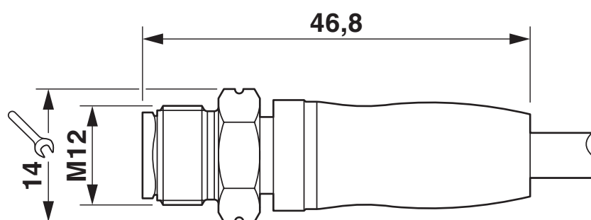
Dessin coté
