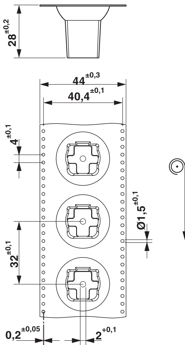
Dessin coté
