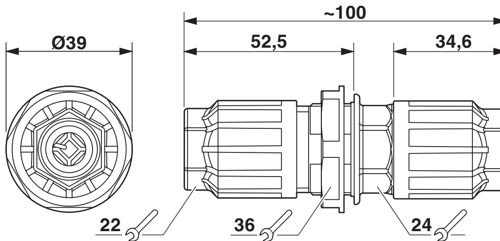
Dessin coté
