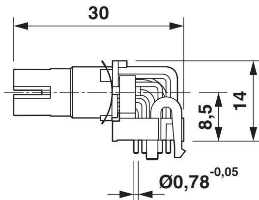
Dessin coté
