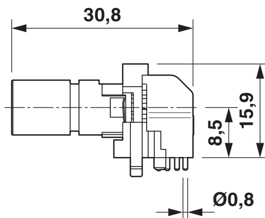
Dessin coté
