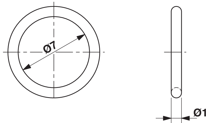
Dessin coté
