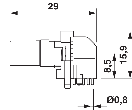
Dessin coté
