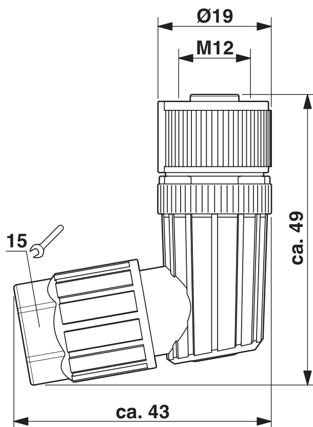
Dessin coté
