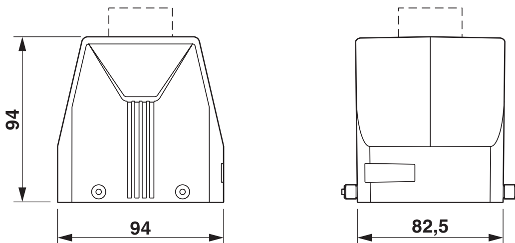
Dessin coté
