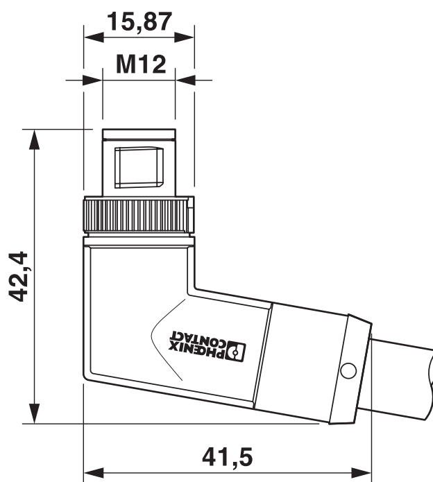
Dessin coté
