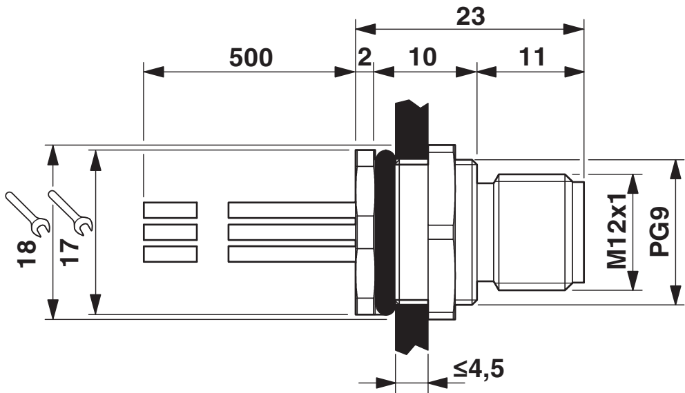
Dessin coté
