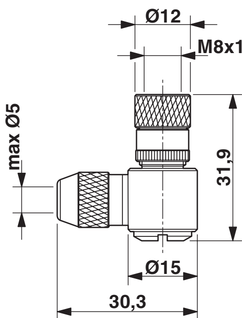
Dessin coté
