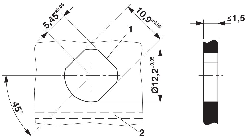
Dessin coté
