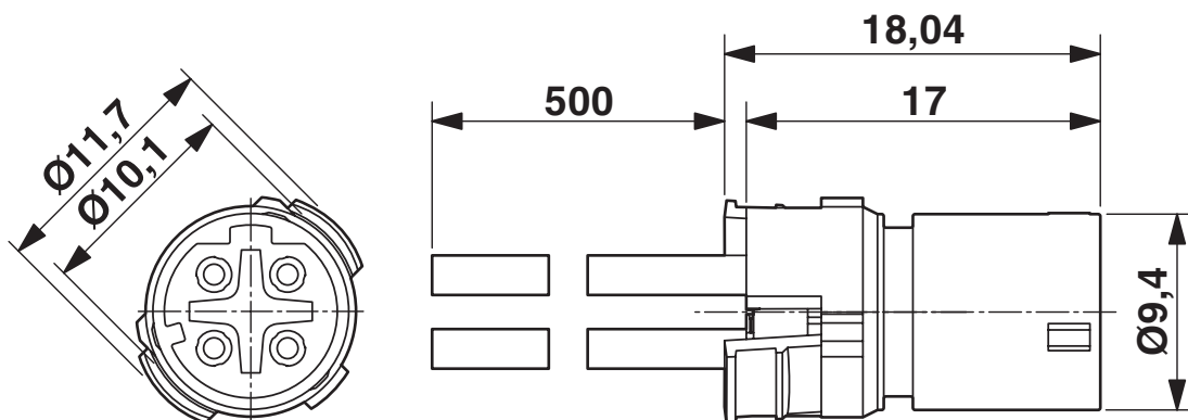
Dessin coté
