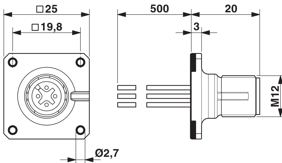
Dessin coté
