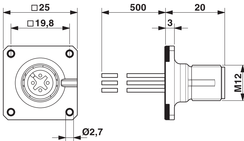
Dessin coté
