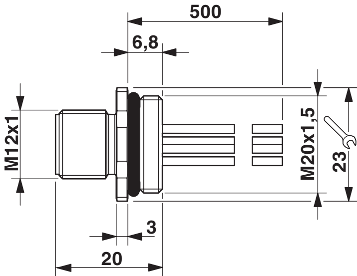
Dessin coté
