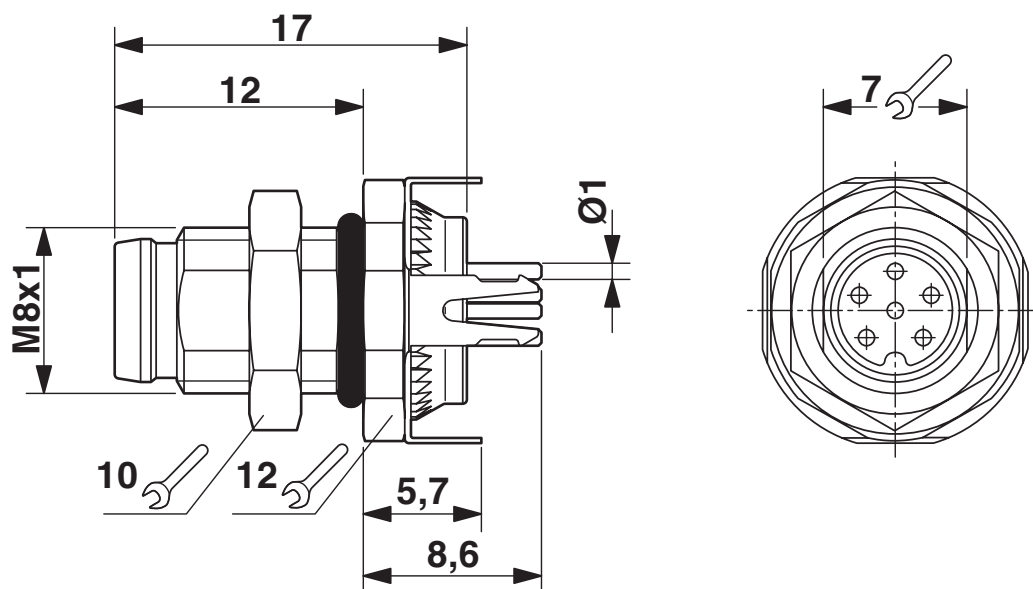
Dessin coté
