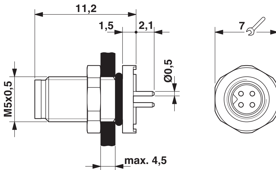
Dessin coté
