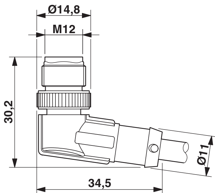
Dessin coté
