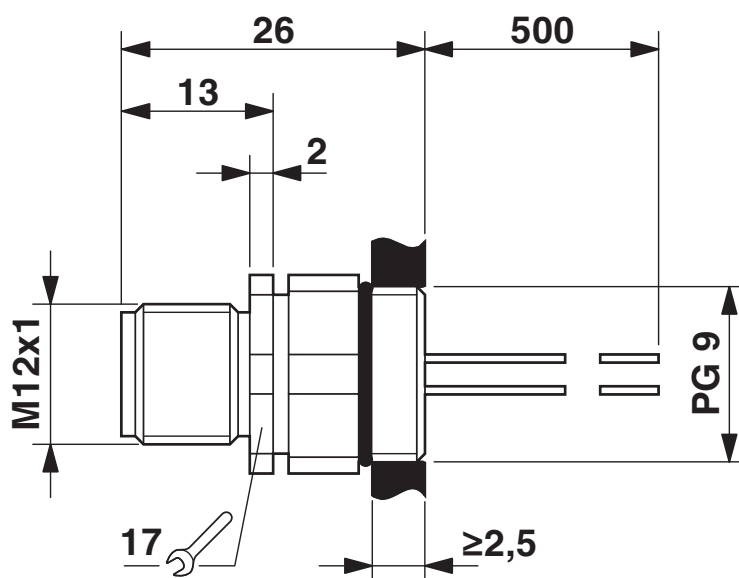
Dessin coté
