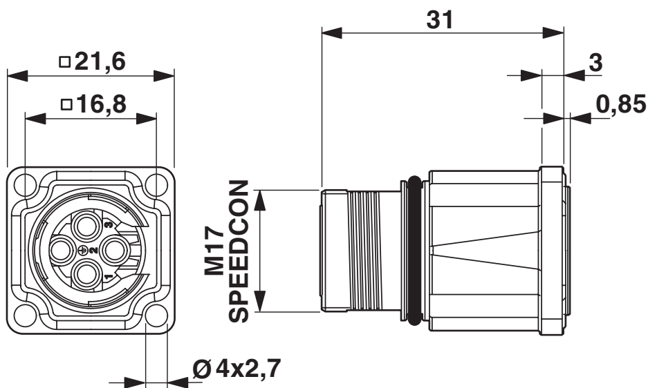
Dessin coté
