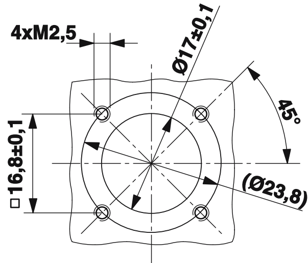
Dessin coté
