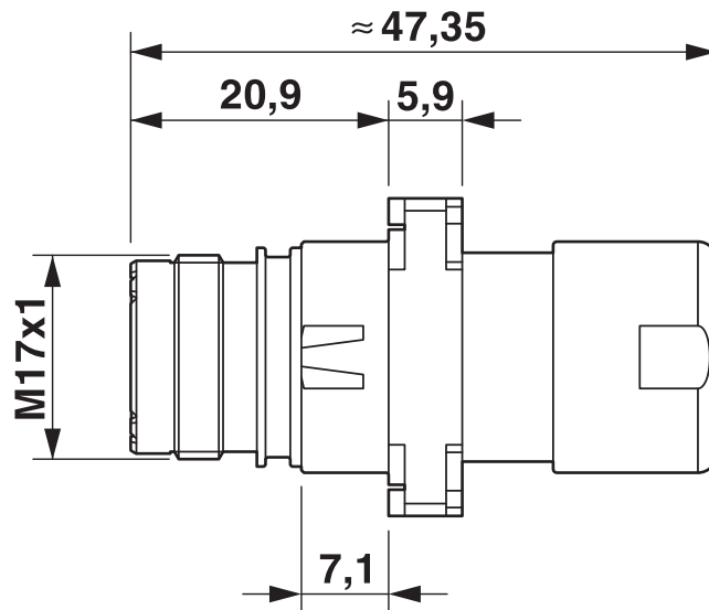
Dessin coté
