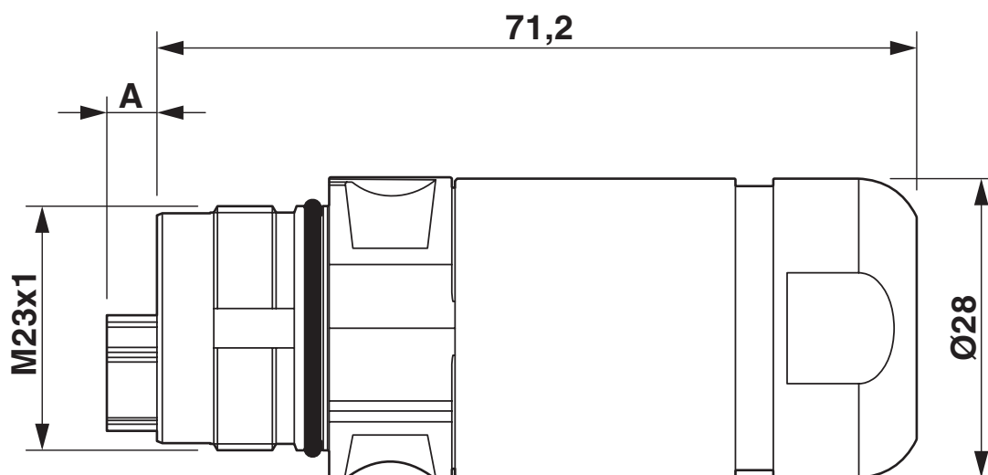
Dessin coté
