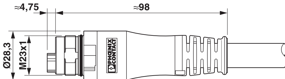
Dessin coté
