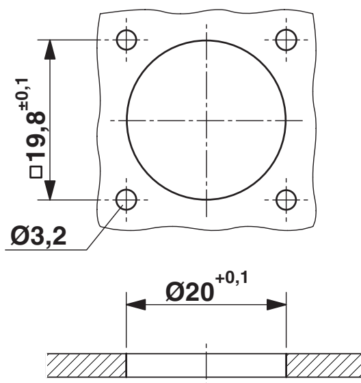
Dessin coté
