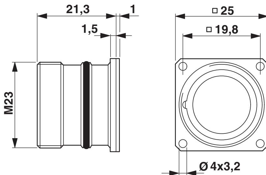
Dessin coté
