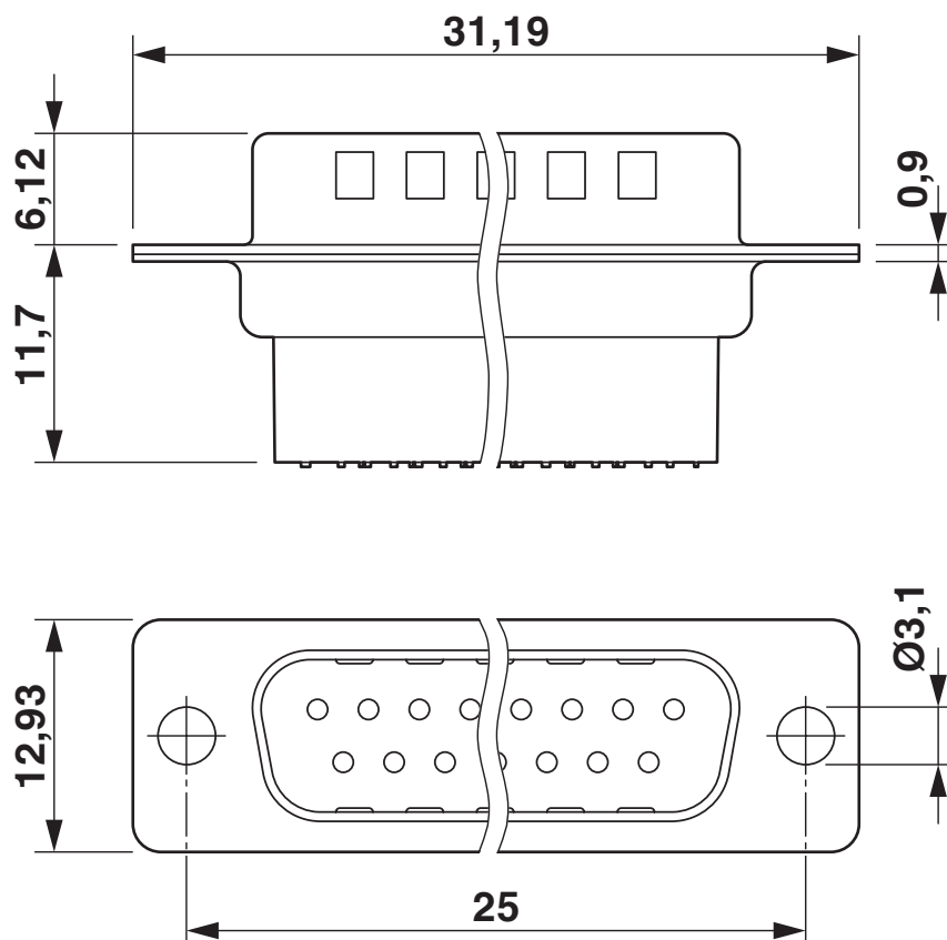
Dessin coté
