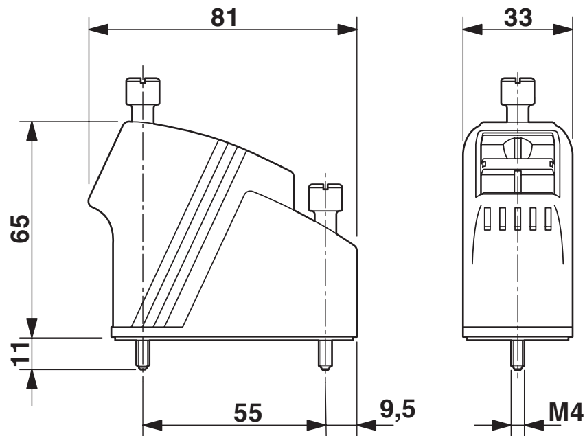
Dessin coté
