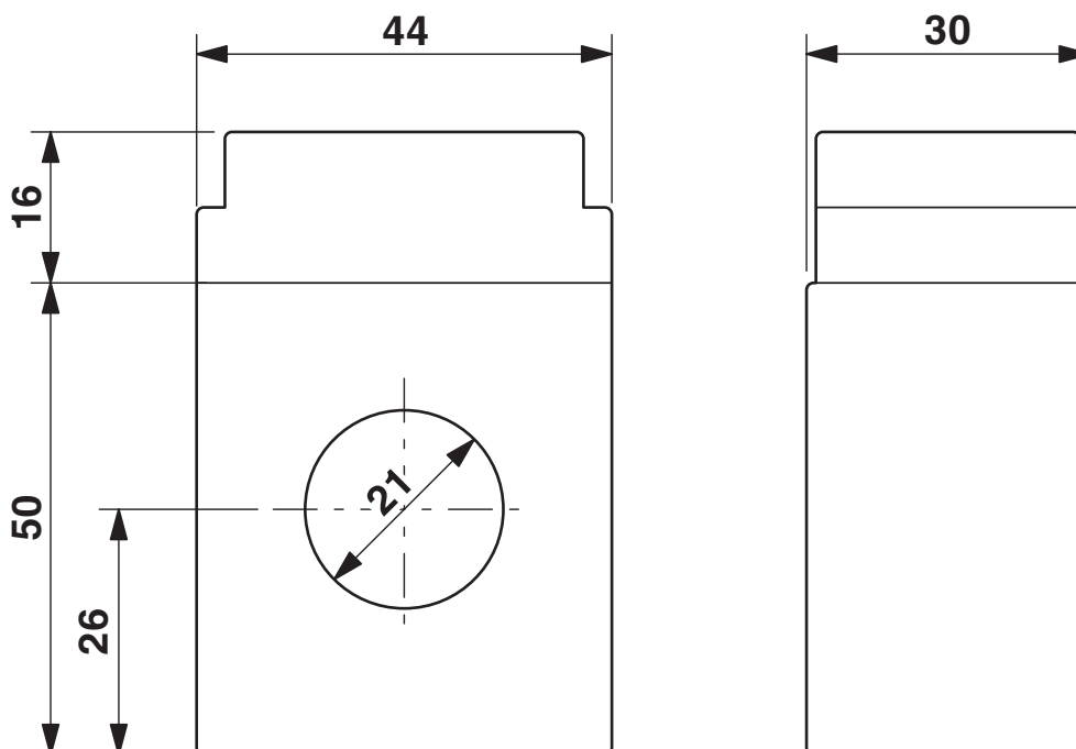
Dessin coté
