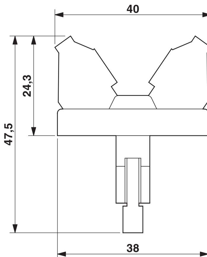
Dessin coté
