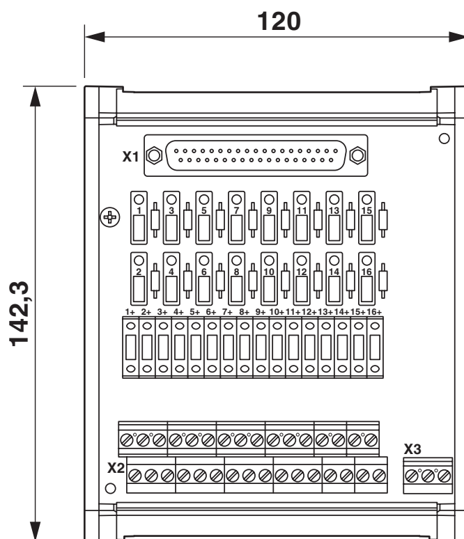
Dessin coté
