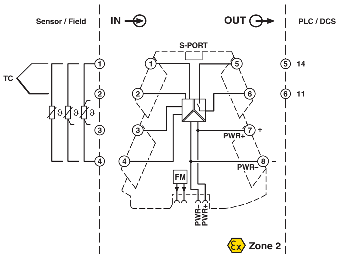
Schéma fonctionnel
