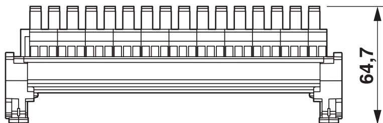
Dessin coté de la version pour droitiers
