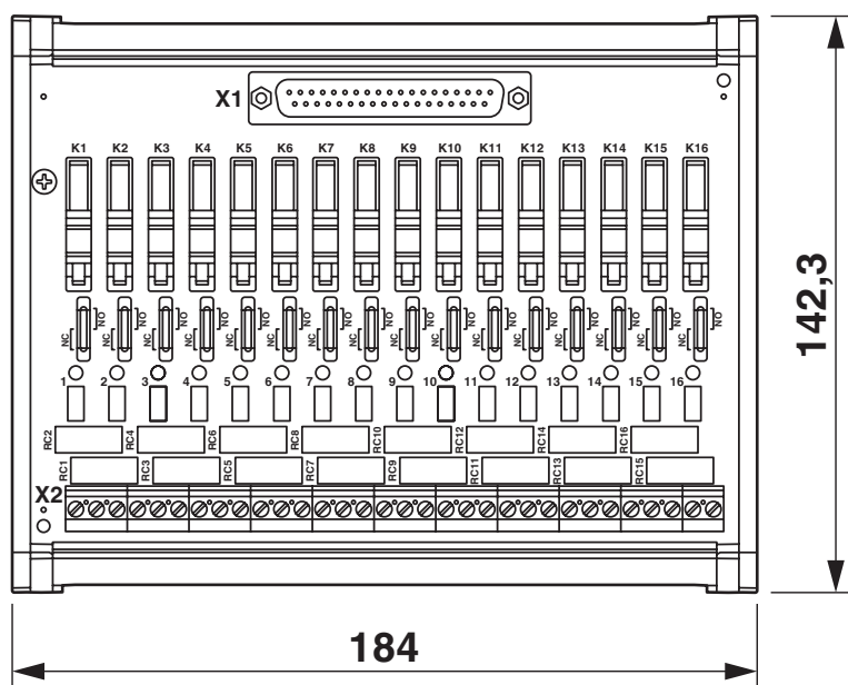
Dessin coté
